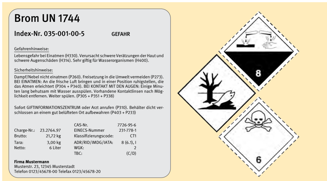
Abbildung 3c: Außenverpackung einer zusammengesetzten Verpackung: Reduziertes Etikett und Gefahrgutkennzeichnung von Brom
