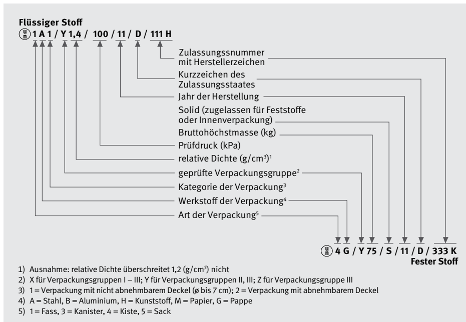
Abbildung 18: Codierung der Verpackungen mit Bauartzulassung
