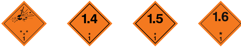
Abbildung 23: Gefahrzettel für explosive Stoffe oder Gegenstände mit Explosivstoff
