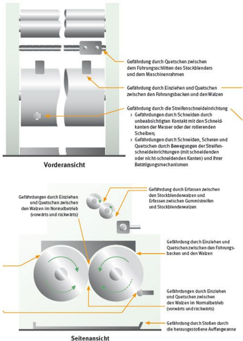
Abbildung 9: Mechanische Gefährdungen an Walzwerken mit Streifenschneideeinrichtung und Stockblender
