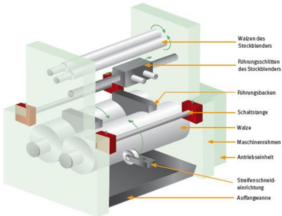
Abbildung 8: Wesentliche Teile eines Walzwerks
