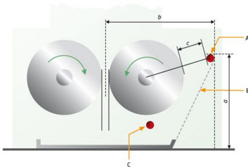
Abbildung 10: Positionierung der Auffangwanne
