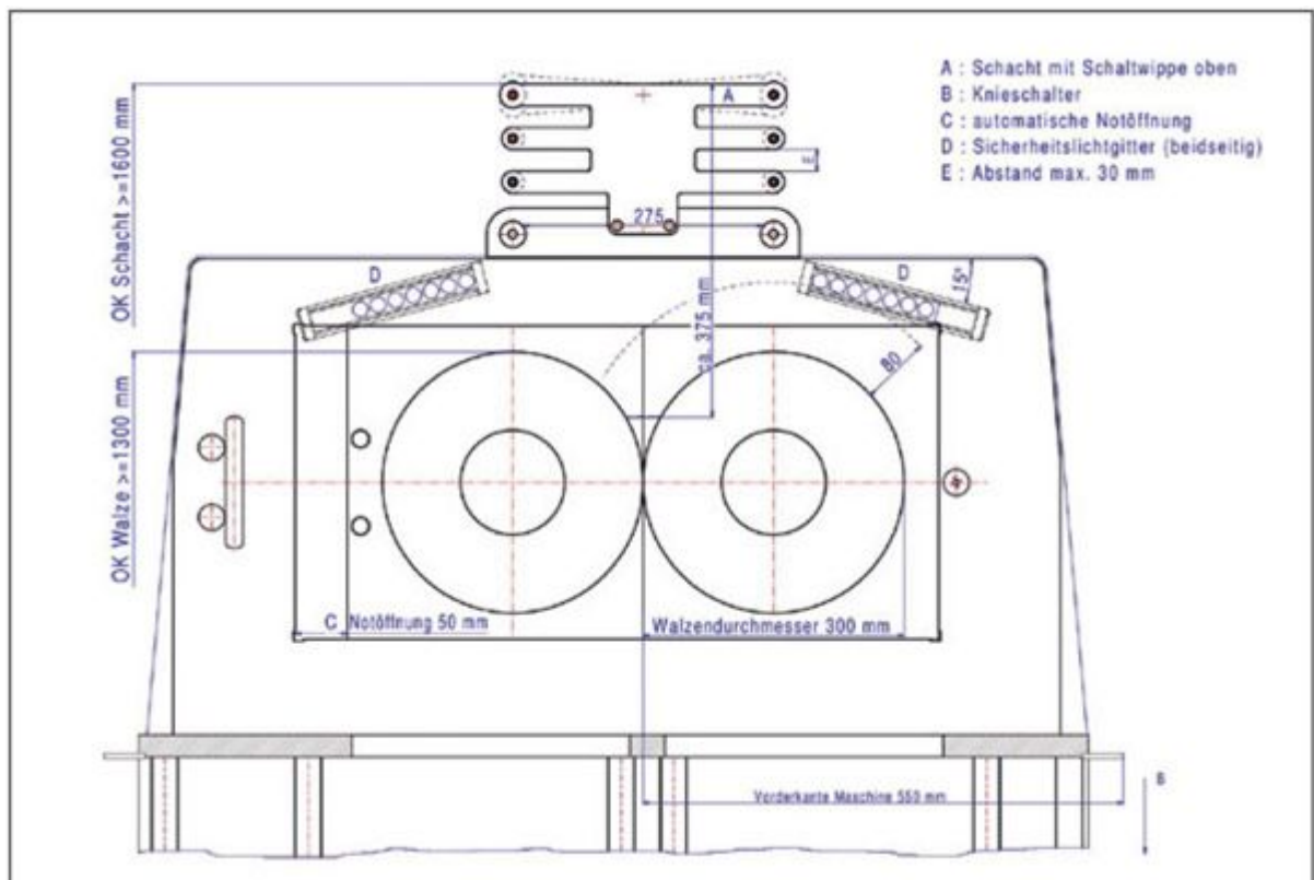
Abbildung 5: Schutzeinrichtung an einem Gummiwalzwerk
