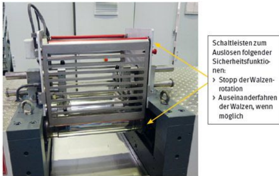
Abbildung 4: Nachgerüstete Schutzeinrichtung an einem Laborwalzwerk (Baujahr vor 1995)
