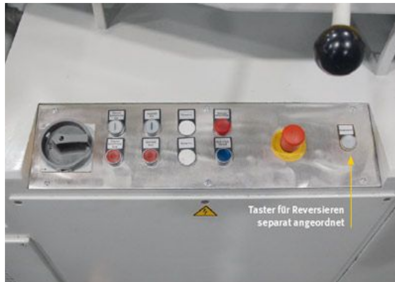
Abbildung 16: Reversieren auf Anforderung nach Not-Halt
