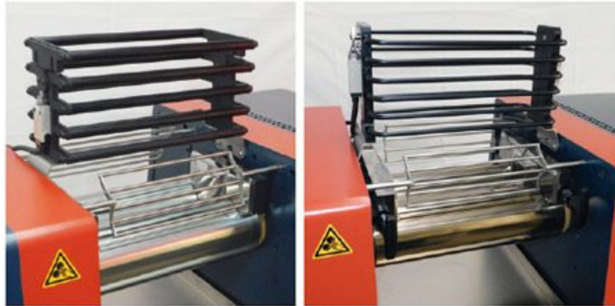
Abbildung 3: Schutzeinrichtungen an einem Laborwalzwerk
