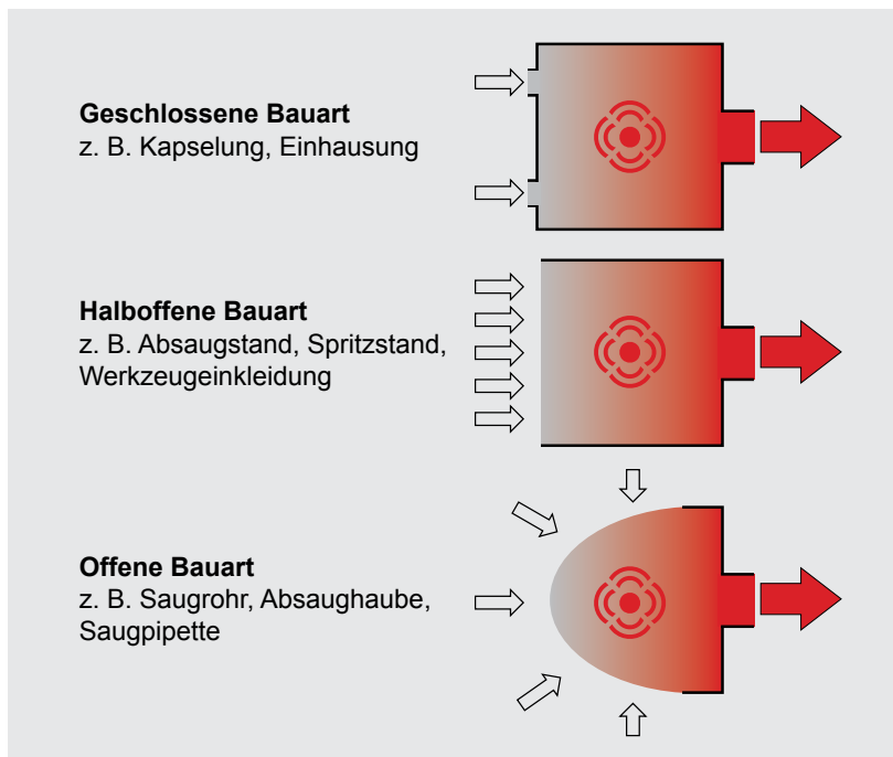
105 Abbildung 7: Bauarten von Erfassungseinrichtungen (Quelle mit Emissionen rot, Zuluft blau)
