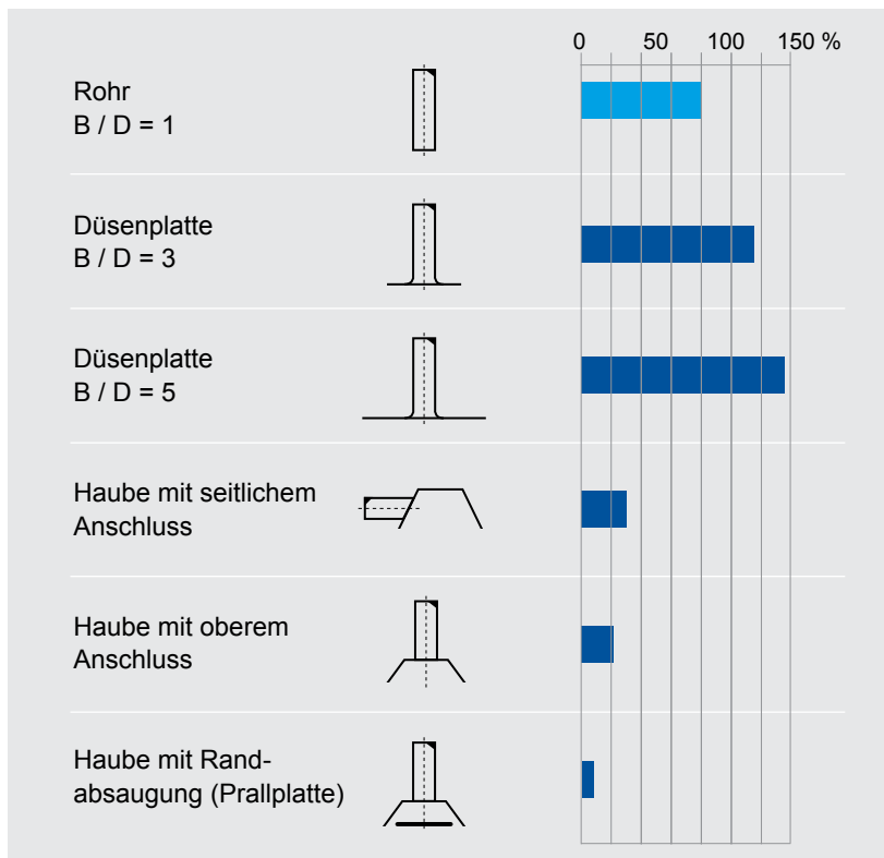
127 133 Abbildung 8: Gütegrad von Erfassungseinrichtungen (B – Breite der Erfassungseinrichtung, D – Durchmesser des Saugrohrs). Zum Vergleich der Gütegrade wurde der des Rohrs als Referenz auf 100 % gesetzt.
