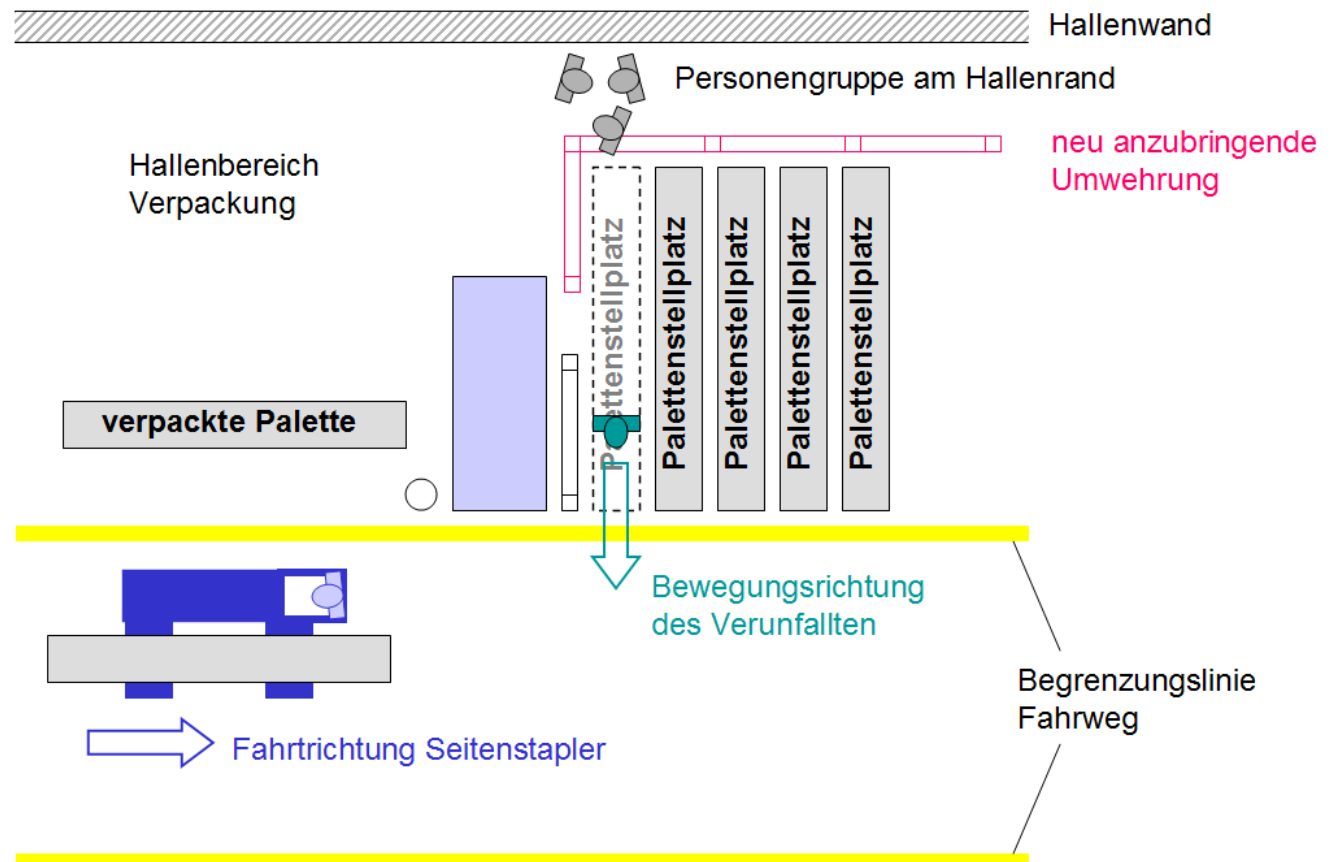
Skizze eines Hallenausschnitts in der Draufsicht
